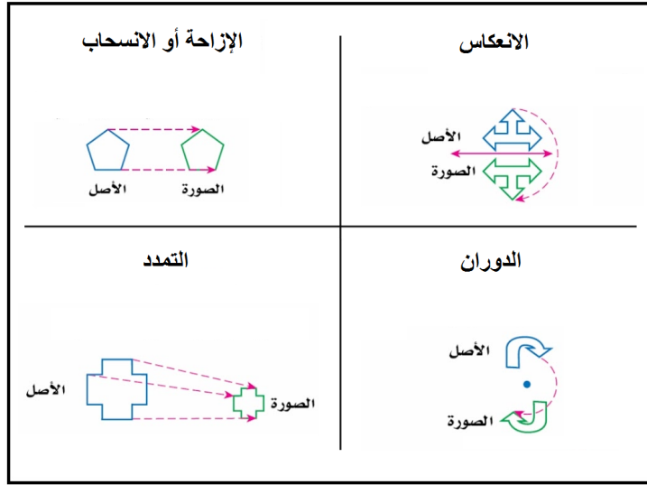
الشكل رقم (3.3): التحويلات الهندسية المحتملة
