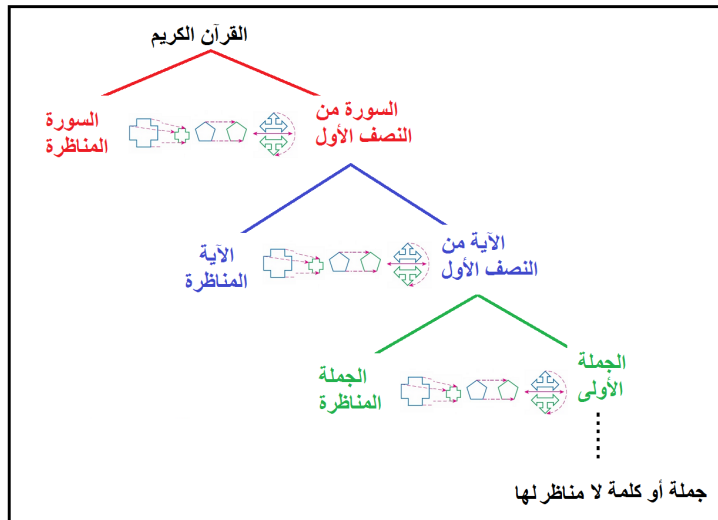
الشكل رقم (3.4): مستويات التناظر
